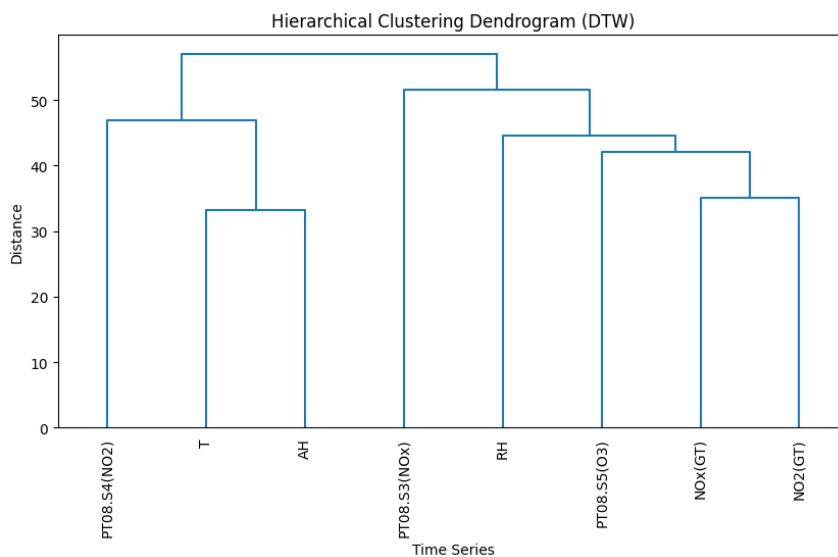
Слика 26. Дендрограм визуализација на кластери добиени со HC
